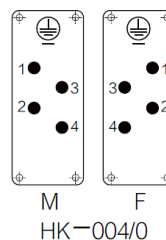
Расположение контактов со стороны соединения
